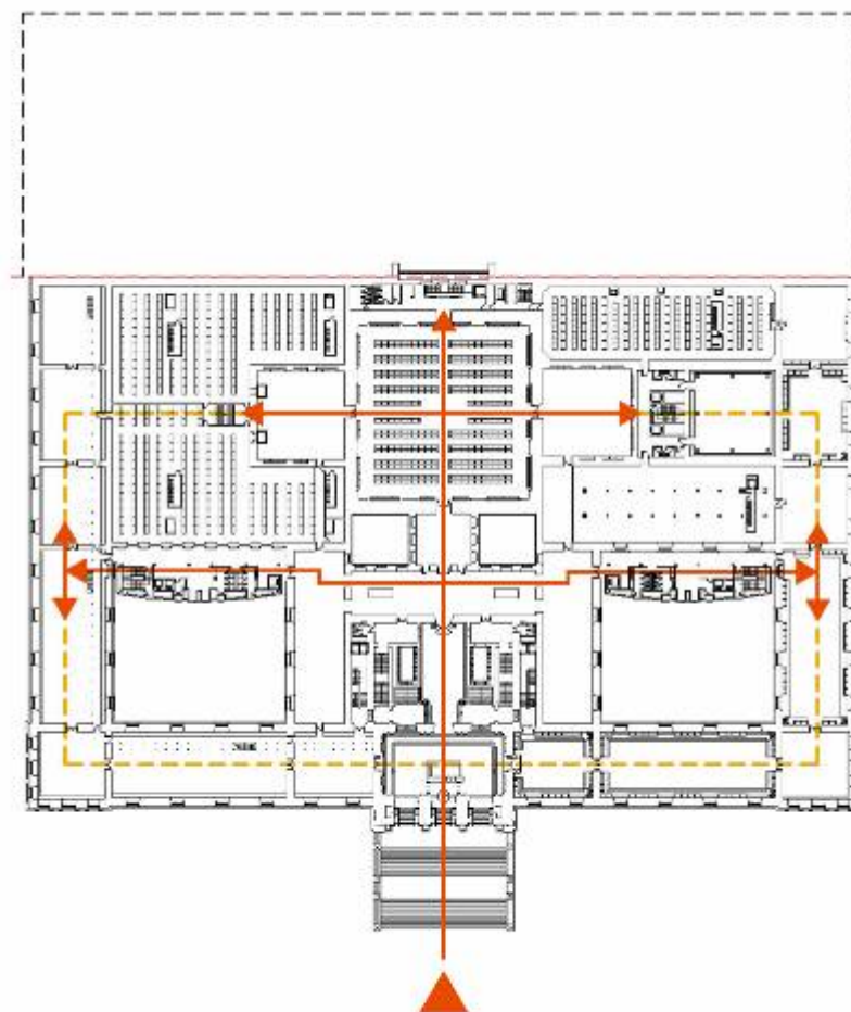
Esquema funcional en anillo
