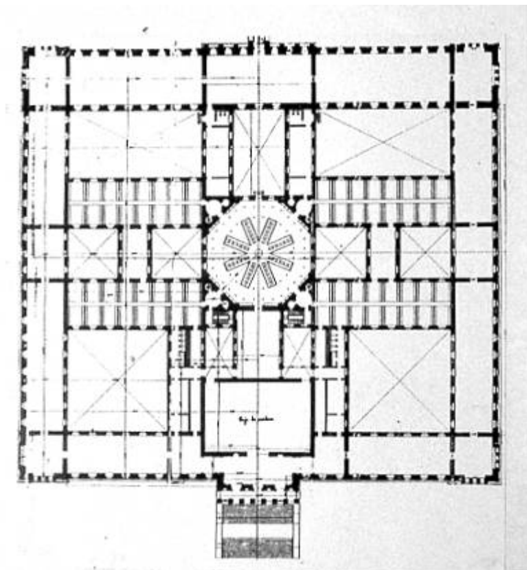
Planta de Jareño
