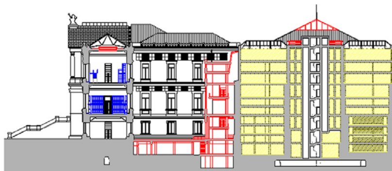
SECCIÓN TRANSVERSAL 1-1
