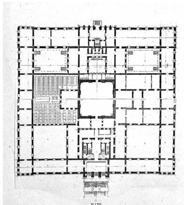
Planta de Ruiz de Salces
