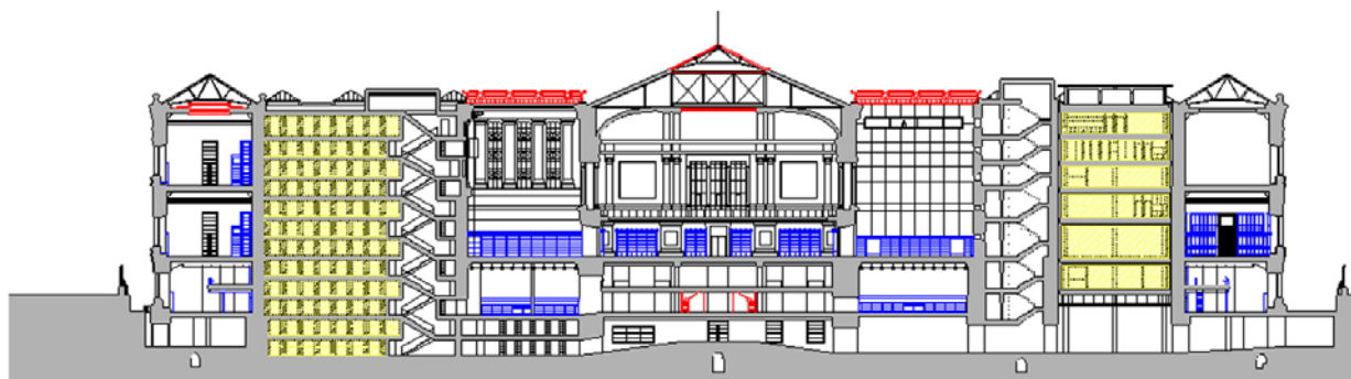
SECCION LONGITUDINAL A-A
