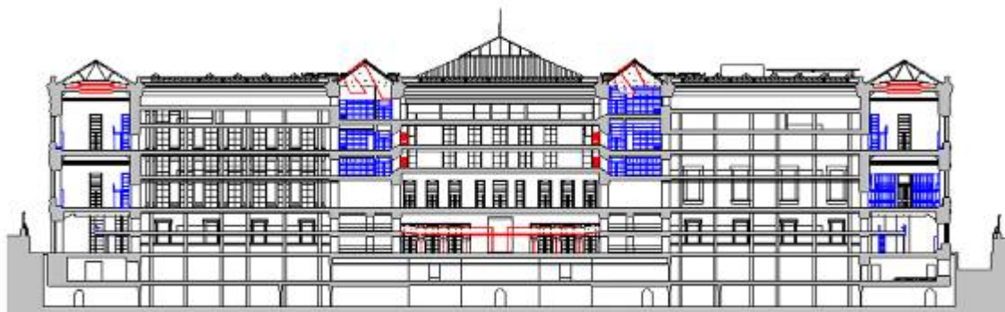
SECCION LONGITUDINAL, D-D
